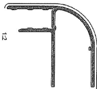
Dachgurtprofil 98*88mm mit 20 und 41mm Aufnahme
