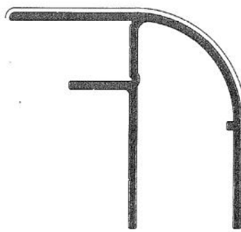
Dachgurtprofil 98*88mm mit 25 und 41mm Aufnahme
