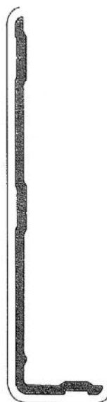
Sockelleiste—Scheuerleiste 110/30 * 2,5 mm
