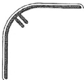
Außen-Eckprofil 100*100*3mm
