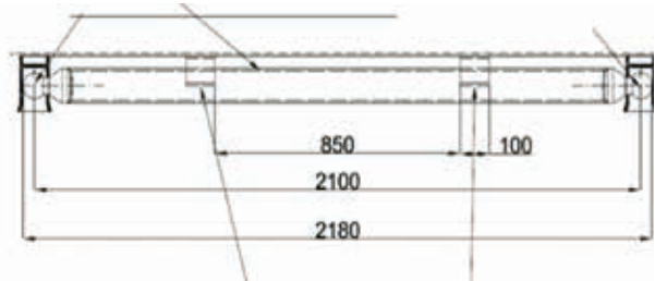
Hinter Kippwelle mit 80er Kippkugeln
